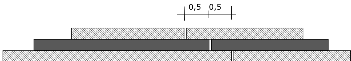
Figuur 1: Verspringende naden bij meerdere asfaltlagen.
